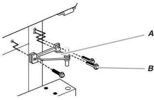
A. Bisagra central B. Tornillos de cabeza hexagonal de la bisagra de \frac{5}{16} "
