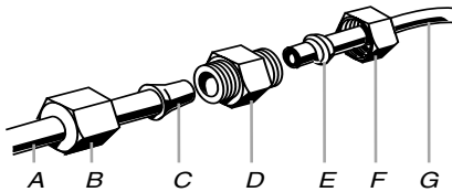
A. Tubería de agua D. Acoplamiento (provisto) B. Tuerca (provista) E. Férula (adquirida) C. Bulbo F. Tuerca (adquirida) G. Tubería de cobre
